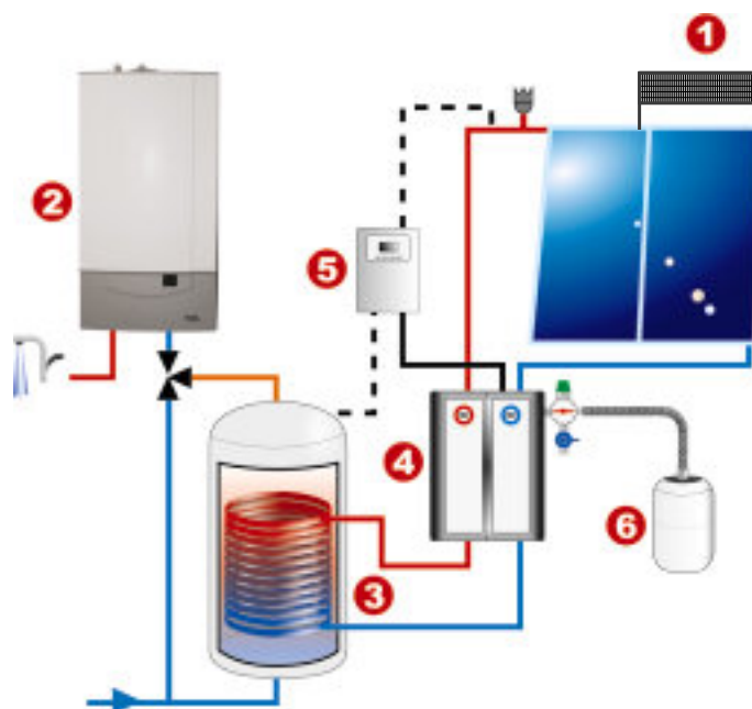
Esempio di impianto solare integrato con caldaia.
