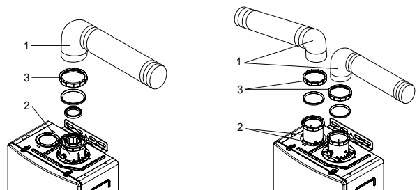
Sistema sdoppiato Ø 80-80
