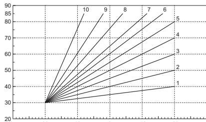
fig. 14 - Curve di compensazione
