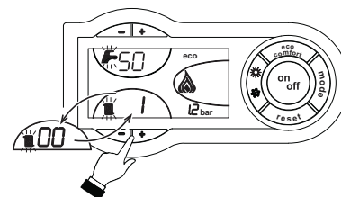
fig. 25 - Modalità TEST (potenza riscaldamento = 100%)
