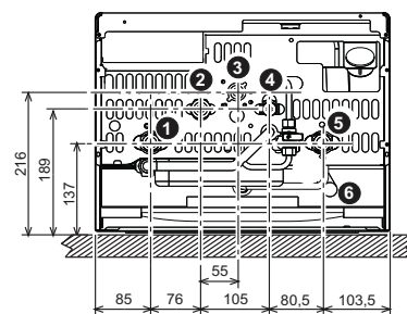
fig. 17 - Attacchi idraulici
