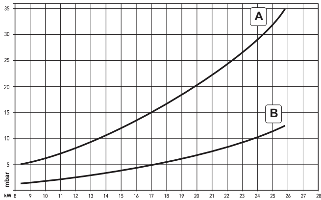
fig. 31 - Diagramma pressione/potenza DIVAtop MICRO LN F 24
