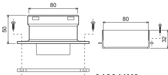
fig. 23 - Accessorio di partenza per condotti separati
