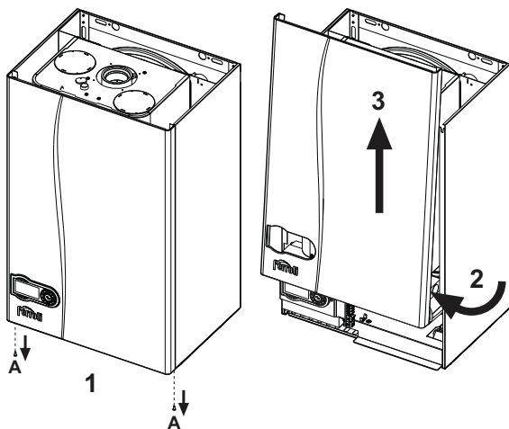
fig. 27 - Apertura mantello
