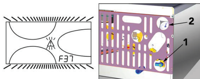
fig. 16 - Anomalia pressione impianto insufficiente
