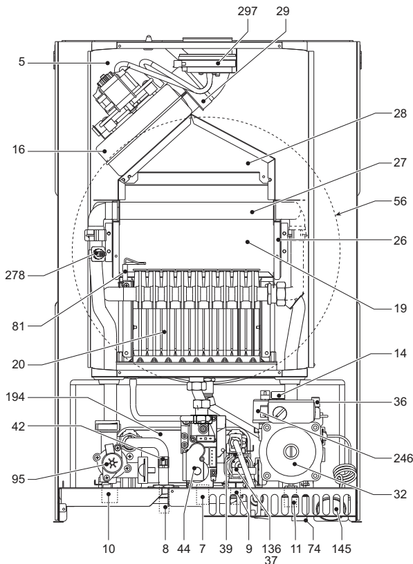
fig. 29 - Vista generale DIVAtop MICRO LN F 24
