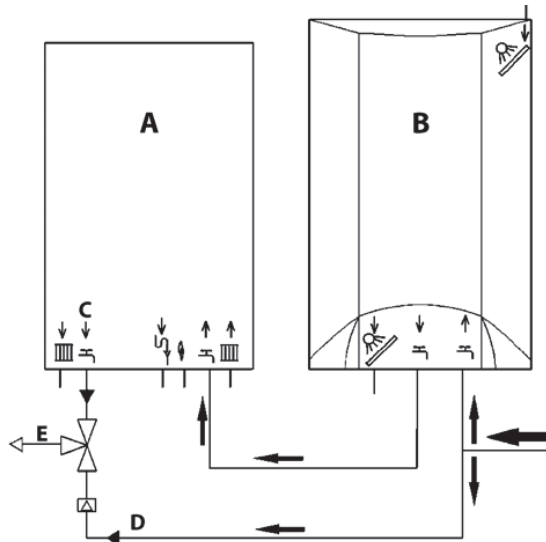
fig. 18 - Schema impianto solare
