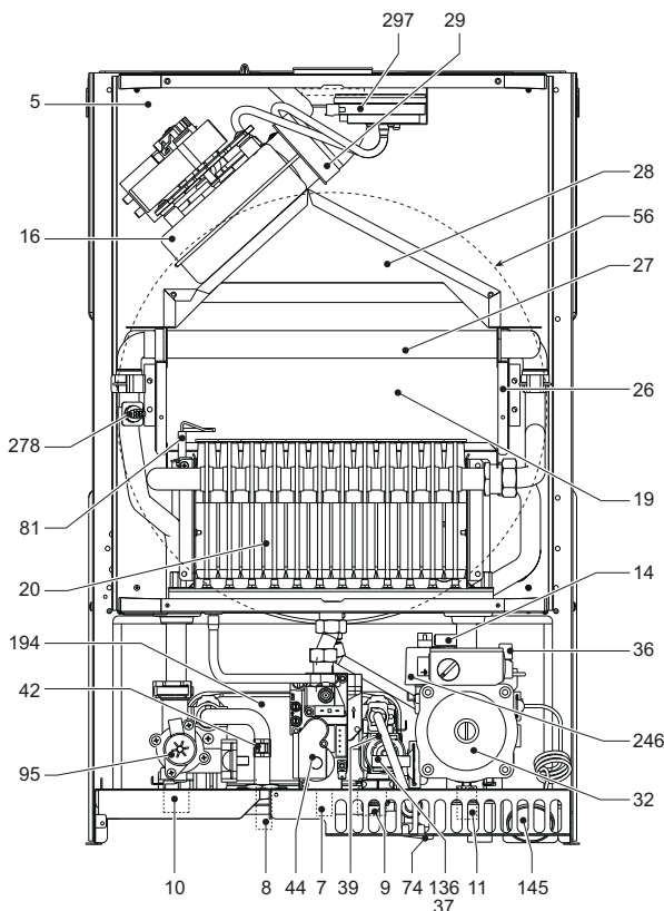
fig. 30 - Vista generale DIVAtop MICRO LN F 32
