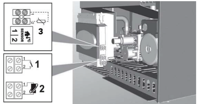
fig. 19 - Accesso alla morsettiera
