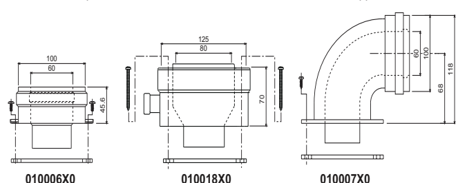
fig. 21 - Accessori di partenza per condotti coassiali
