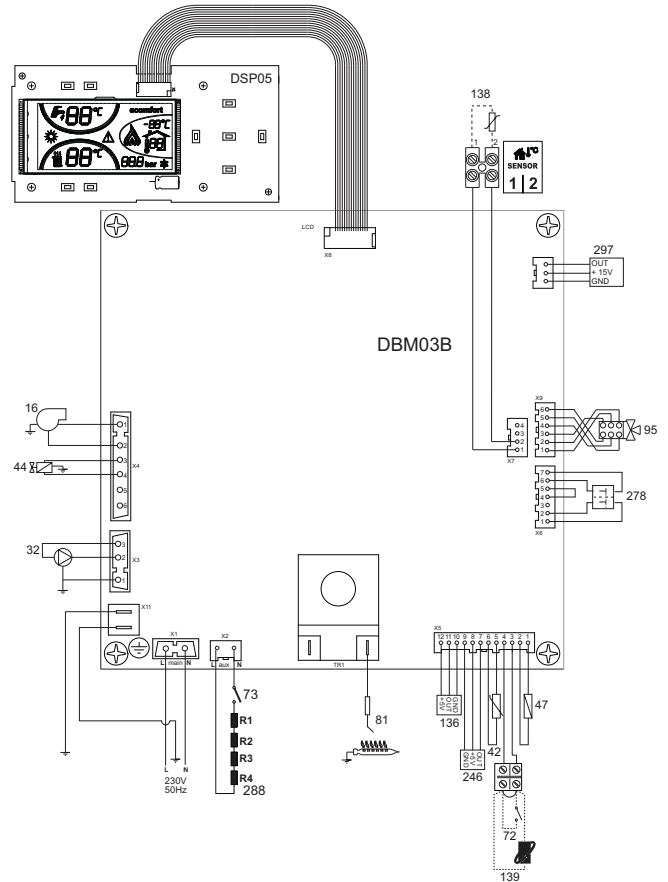
fig. 35 - Schema elettrico
