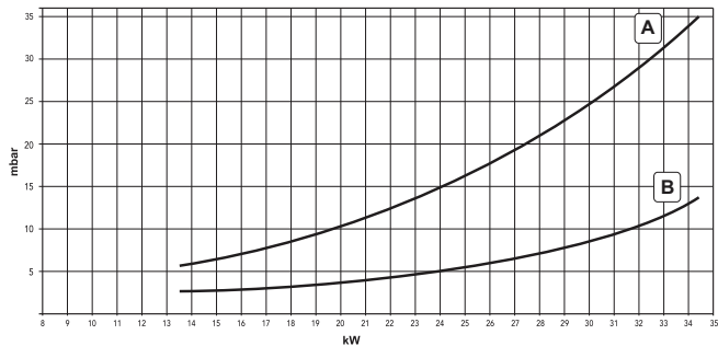
fig. 33 - Diagramma pressione/potenza DIVAtop MICRO LN F 32
