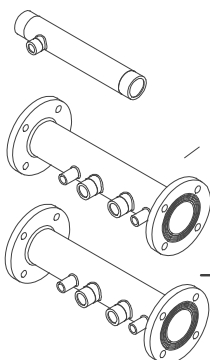
Kit collettori mandata-ritorno-gas per caldaia singola
