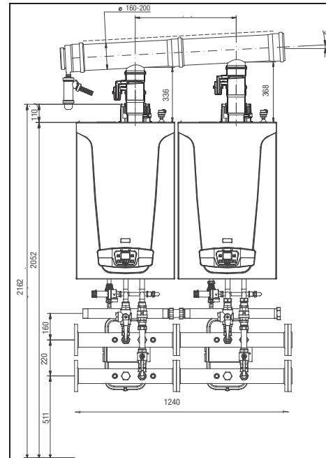
Condensy A 100 RSE
