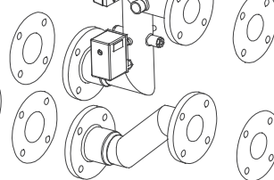
Kit idraulico collettore ISPESL per separatore idraulico
