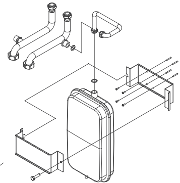
Kit collegamento vaso espansione
