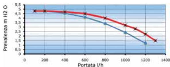
Bolli 128 SE Portata/Prevalenza alla placca
