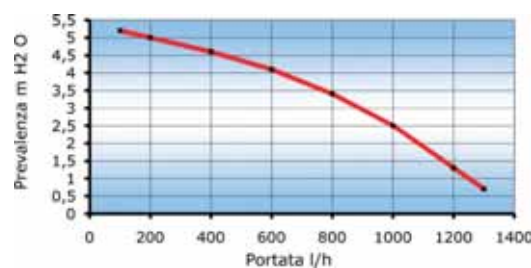
Ester white 24 SE Portata/Prevalenza alla placca
