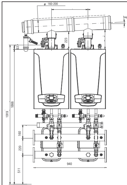
Condensy A 55 RSE
