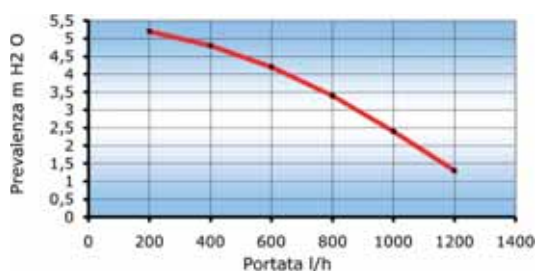
Wally Condensy 24 SE Portata/Prevalenza alla placca
