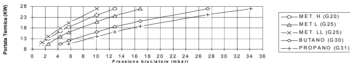
2.12.1 DIAGRAMMA PRESSIONE GAS - PORTATA TERMICA
