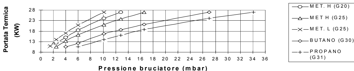
2.13.1 DIAGRAMMA PRESSIONE GAS - PORTATA TERMICA
