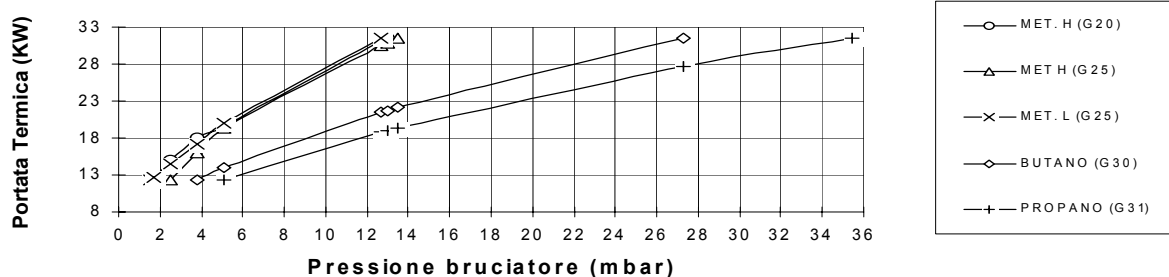
2.14.1 DIAGRAMMA PRESSIONE GAS - PORTATA TERMICA
