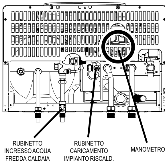
VISTA DAL BASSO DELLA CALDAIA
