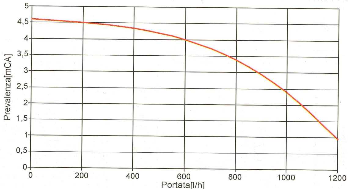
Grafico 1: Prevalenza disponibile all'impianto per CSP SYSTEM TOP serie PLB
