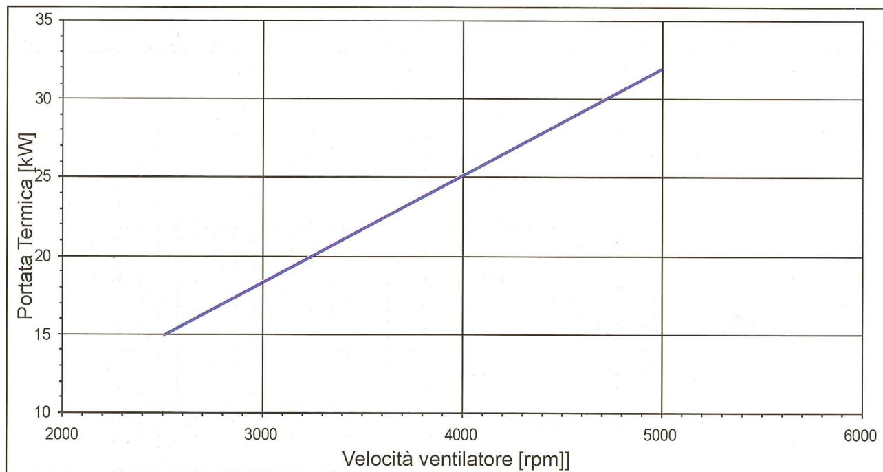
Grafico 8: PORTATA TERMICA
