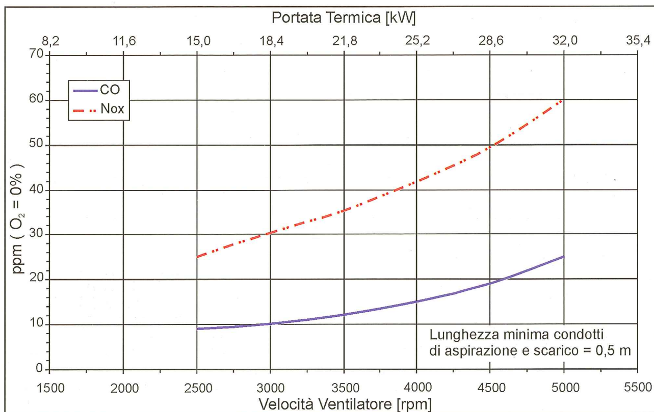
Grafico 4: CURVE CO E NOx (G20)
