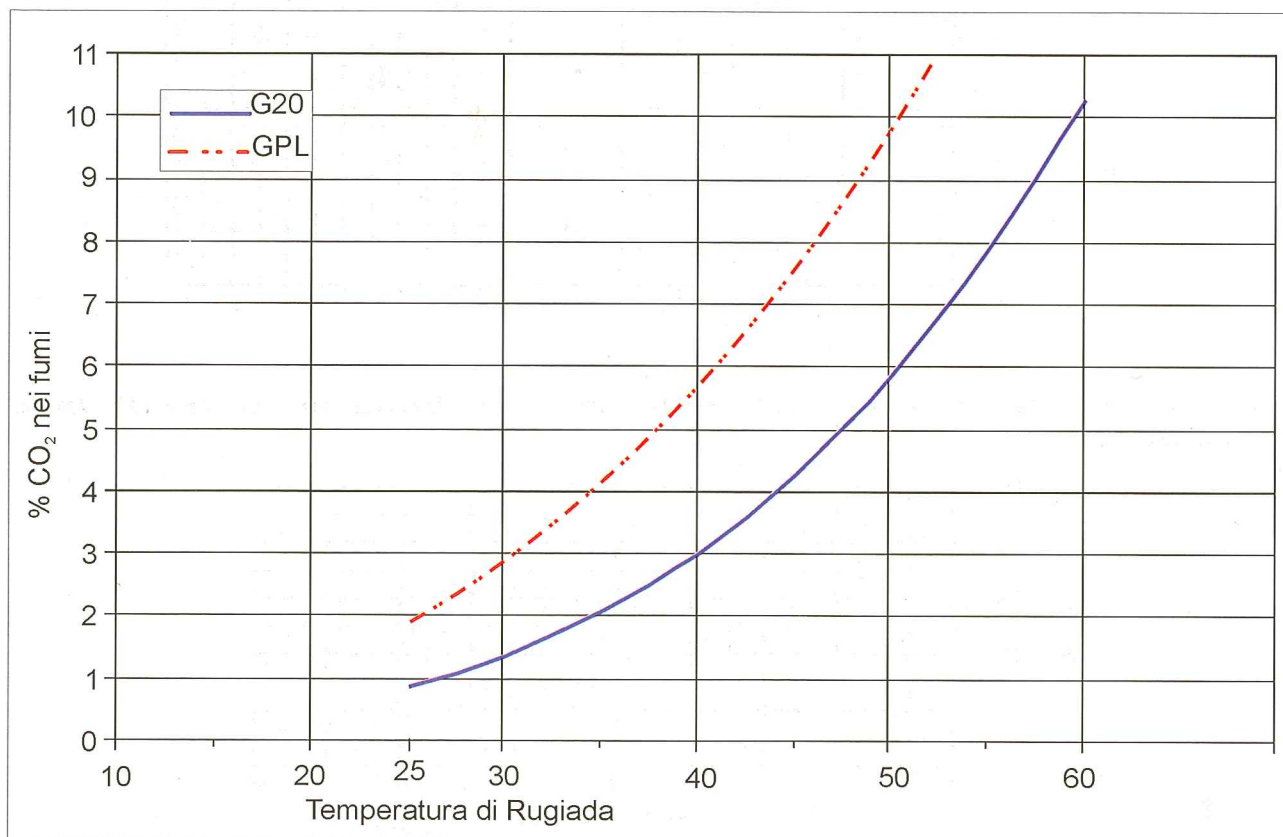
Grafico 9: TEMPERATURA DI RUGIADA
