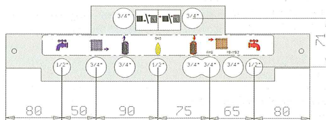
Disegno d'assieme gruppi idraulici
