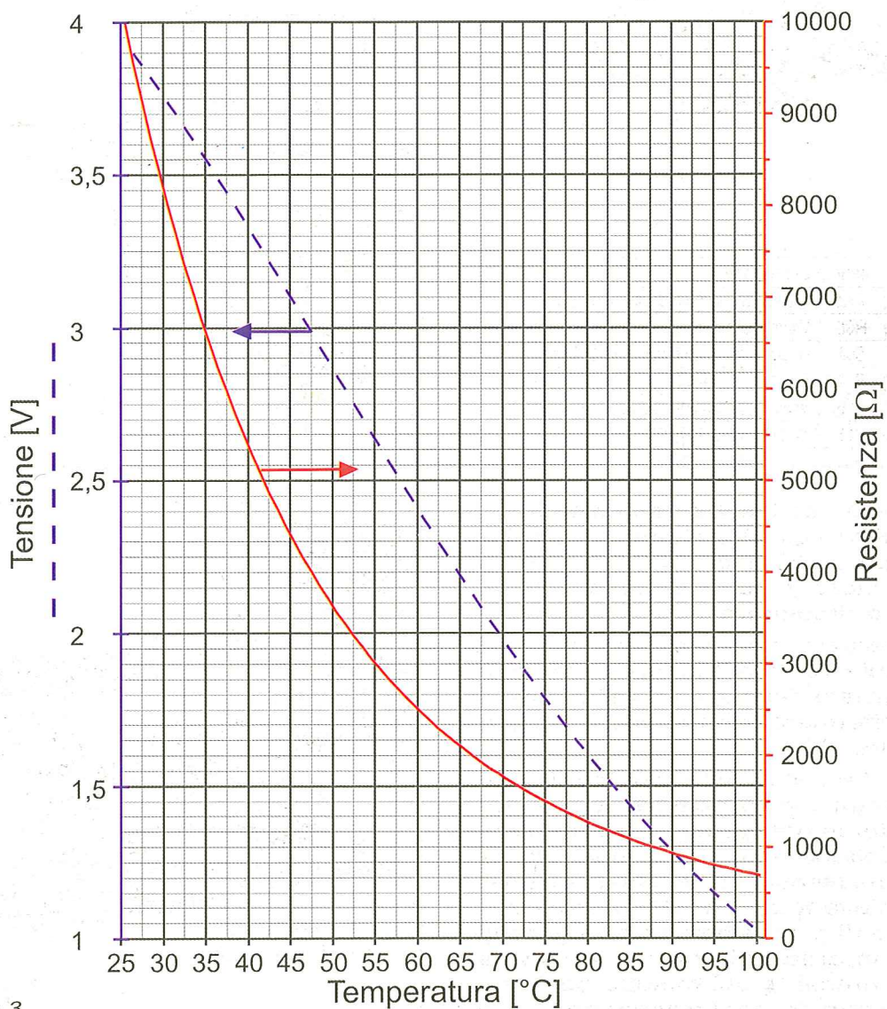
Caratteristiche resistenza elettrica in funzione della temperatura per sonda bollitore compatibili col sistema ALUCOND 500 MB 30
