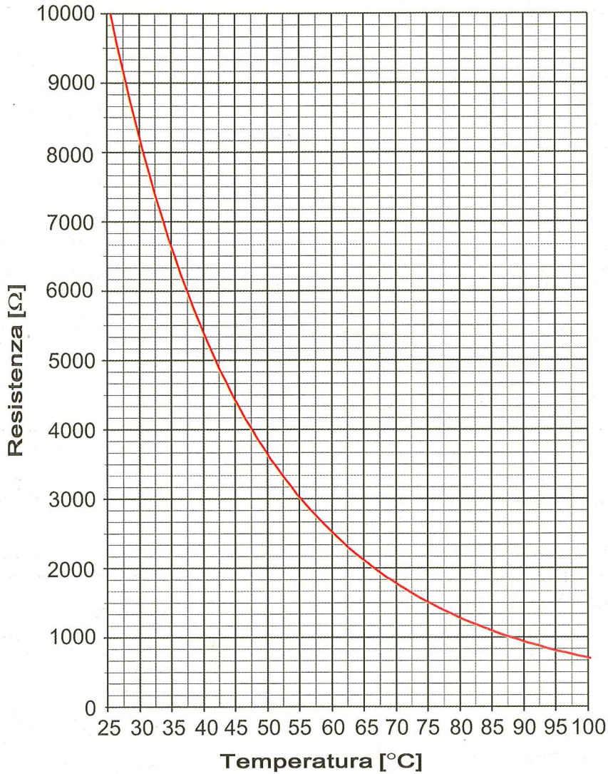
Grafico 5. Valore analogico letto in funzione della temperatura per sonde di temperatura sanitario e riscaldamento
