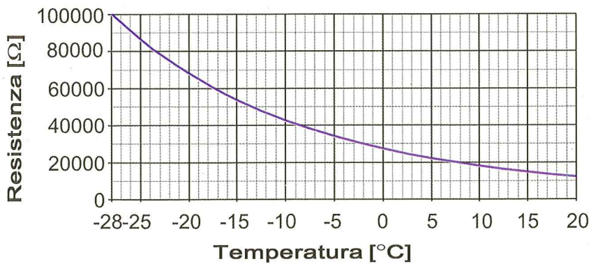
Grafico 6. Valore di resistenza della sonda esterna in funzione della temperatura
