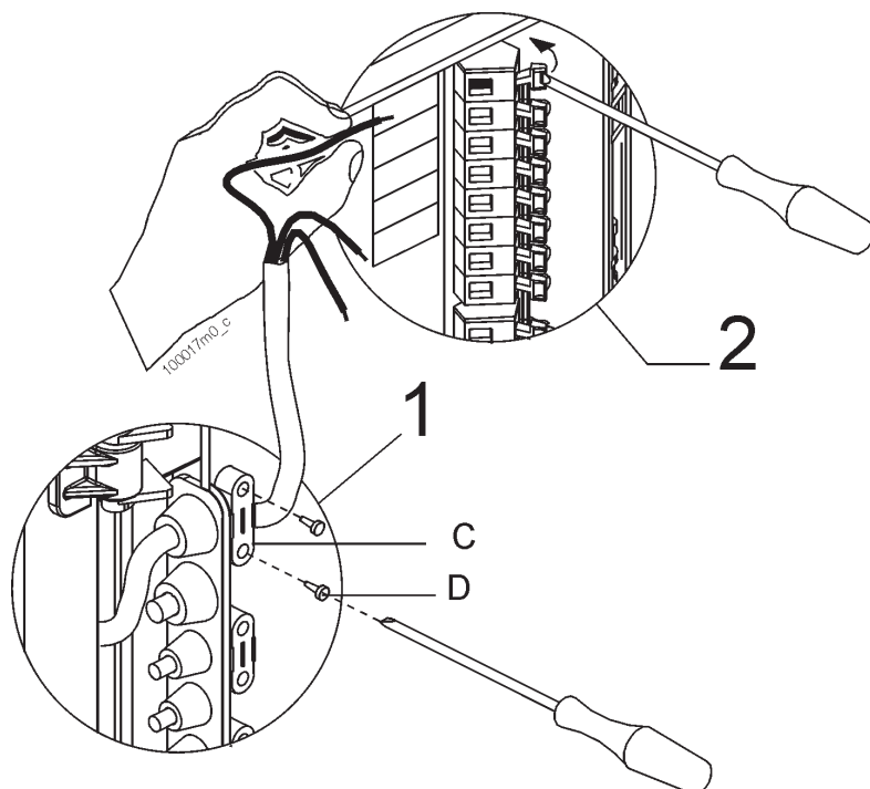
Figura 14 - Collegamento alimentazione
