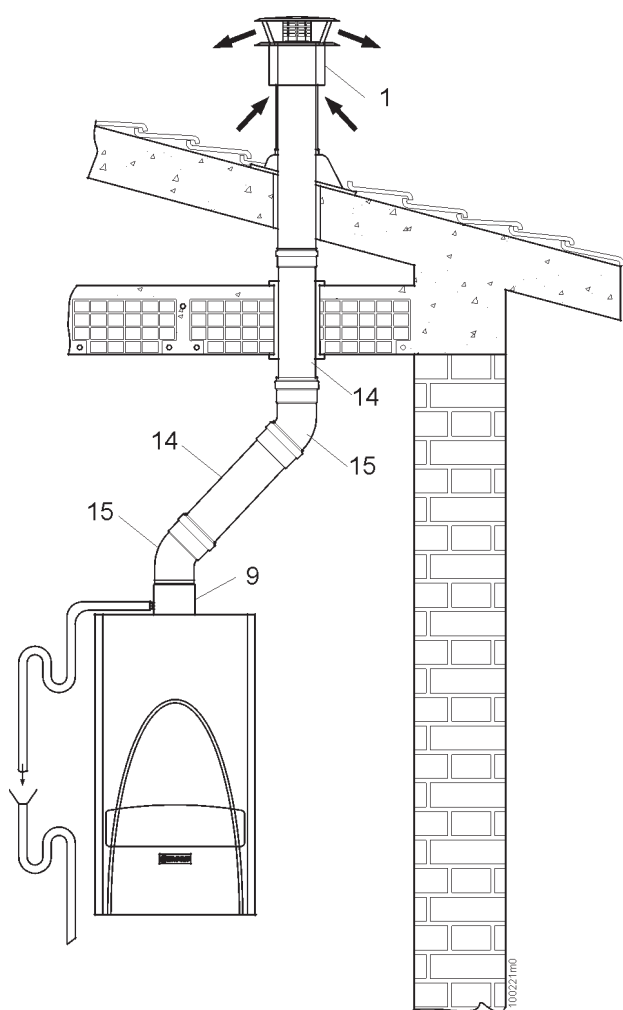
Figura 28 - Esempi di installazione del condotto coassiale
