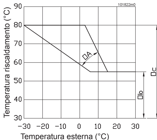
Figura 45 - Grafici riscaldamento con sensore temperatura esterna
