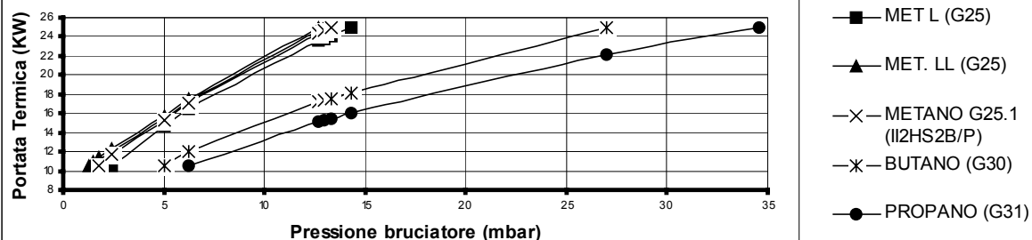
2.10.1 DIAGRAMMA PRESSIONE GAS - PORTATA TERMICA
