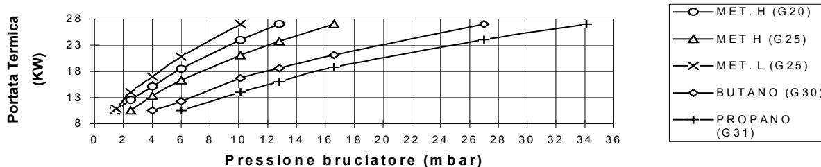
2.12.1 DIAGRAMMA PRESSIONE GAS - PORTATA TERMICA
