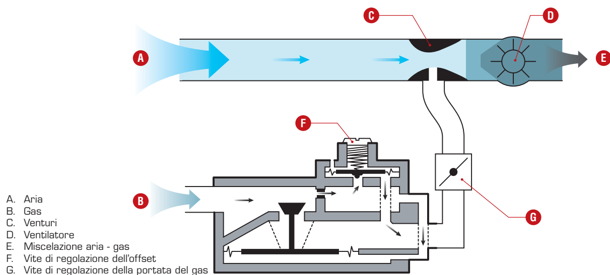
Principio di controllo del miscelatore aria/gas
